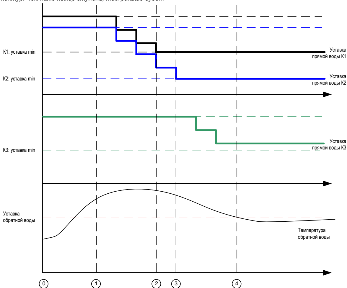
Рис. 17 – Пример работы ограничителя
