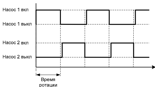
Рис. 14 – Ротация насосов
