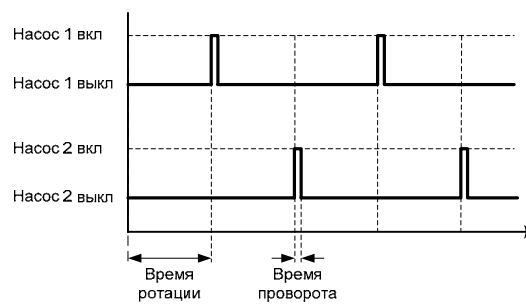
Рис. 15 – Проворот насосов
