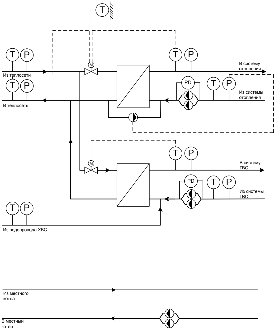
Рис. 1 – Пример схемы автоматизации ИТП
