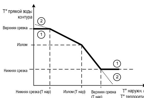
Рис. 16 – Температурный график
