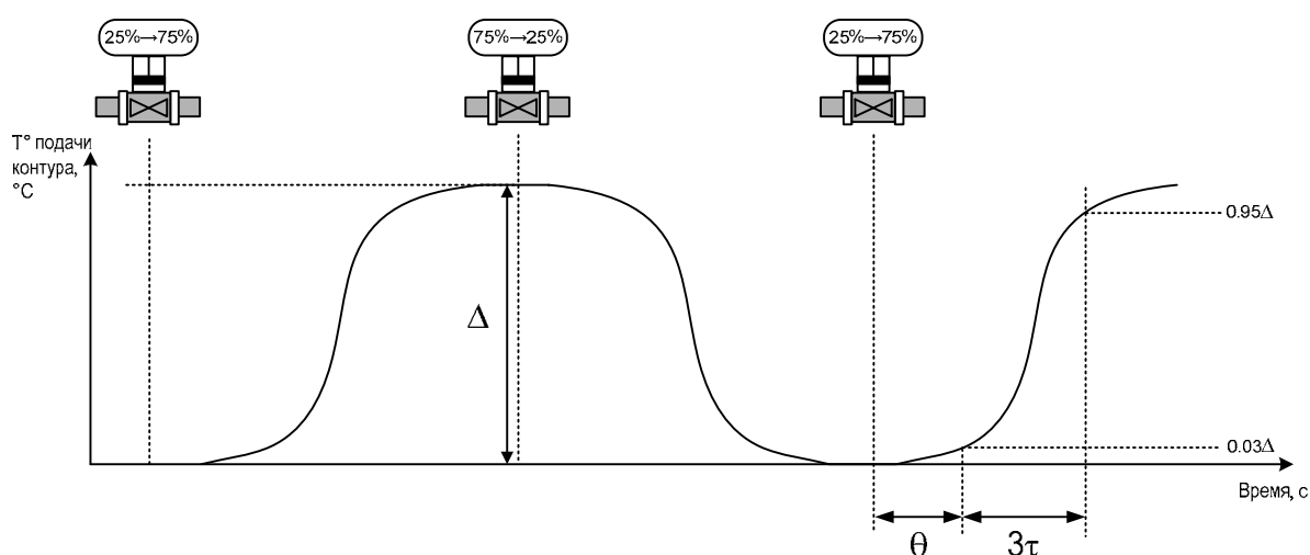
Рис. 19 – Алгоритм настройки регулятора
